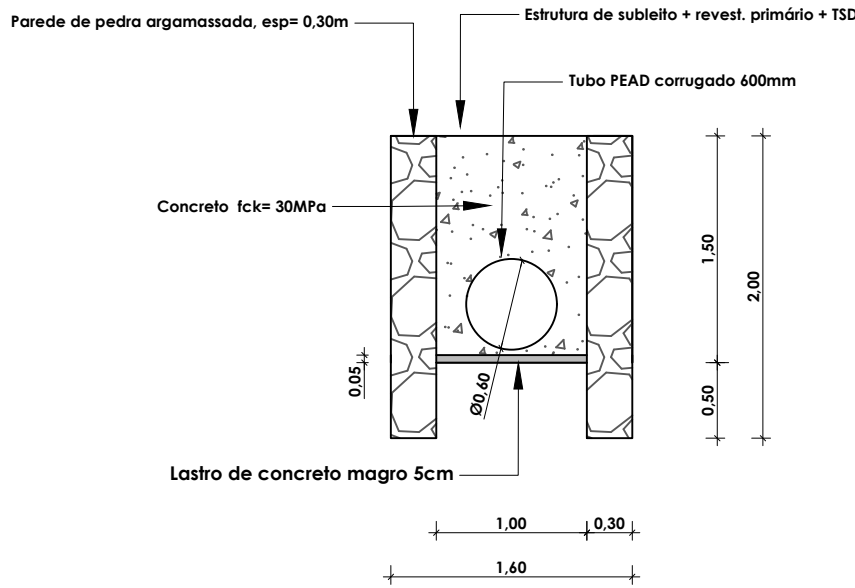
CORTE TRANSVERSAL - DETALHE TUBO PEAD SIMPLES Escala 1/50
