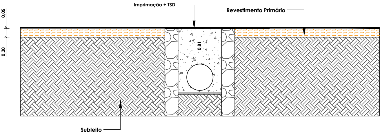
CORTE LONGITUDINAL - PASSAGEM MOLHADA COM PEAD SIMPLES Escala 1/50
